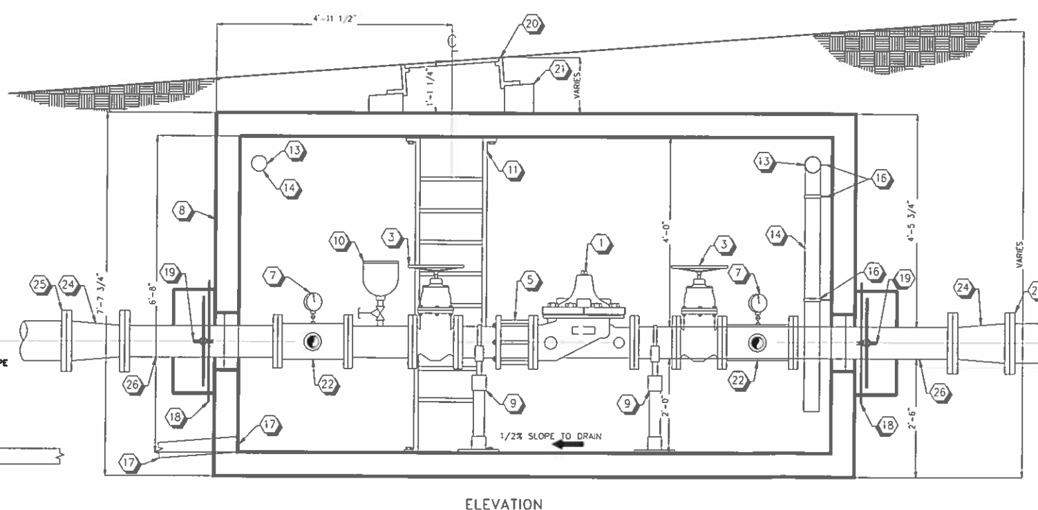
A DETAIL - PRV VAULT TYP N.T.S.
